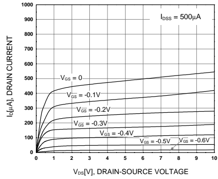
Figure 2. I_D - V_{DS}
