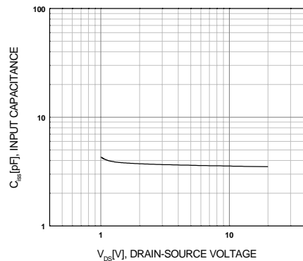
Figure 6. C_{iss} - V_{DS}
