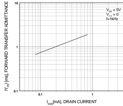
Figure 4. |y_{FS}| - I_{DSS}
