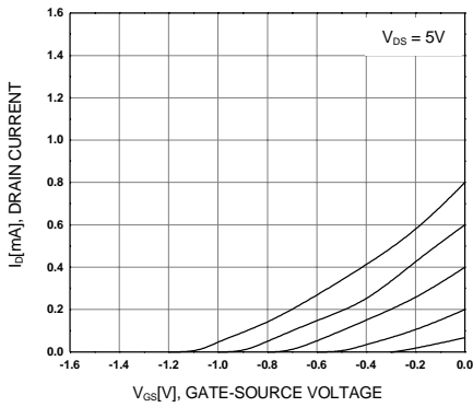
Figure 3. I_D - V_{GS}
