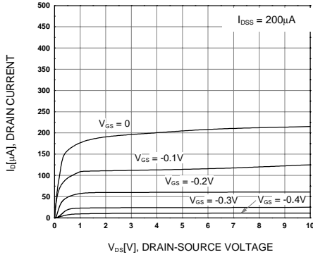
Figure 1. I_D - V_{DS}
