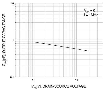
Figure 7. C_{RSS} - V_{DS}
