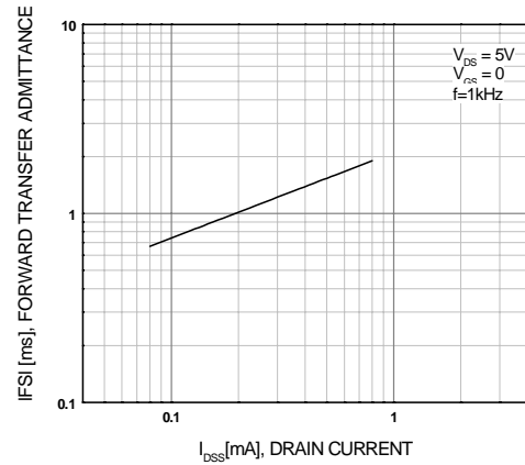
Figure 4. |y_{FS}| - I_{DSS}
