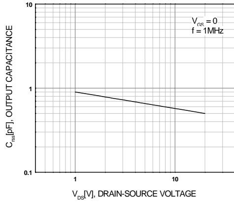
Figure 7. C_{RSS} - V_{DS}
