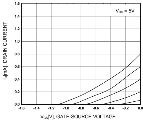
Figure 3. I_D - V_{GS}
