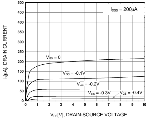
Figure 1. I_D - V_{DS}
