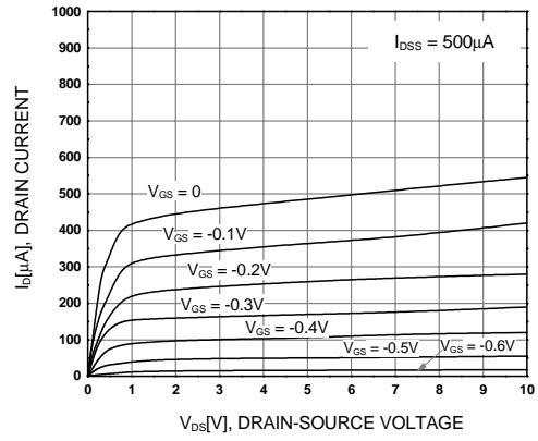
Figure 2. I_D - V_{DS}
