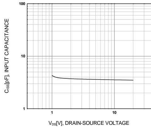
Figure 6. C_{iss} - V_{DS}
