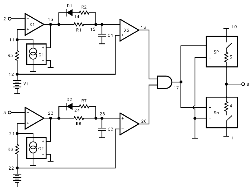
EL7243 Macromodel
