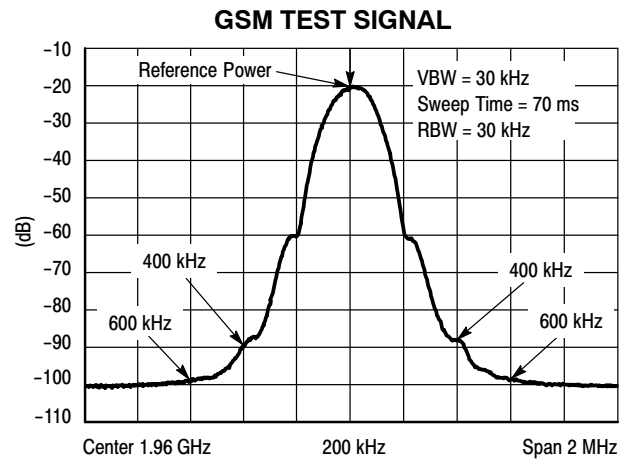
Figure 19. EDGE Spectrum
