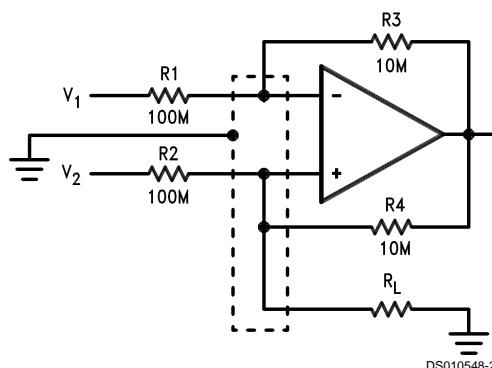
(d) Howland Current Pump
