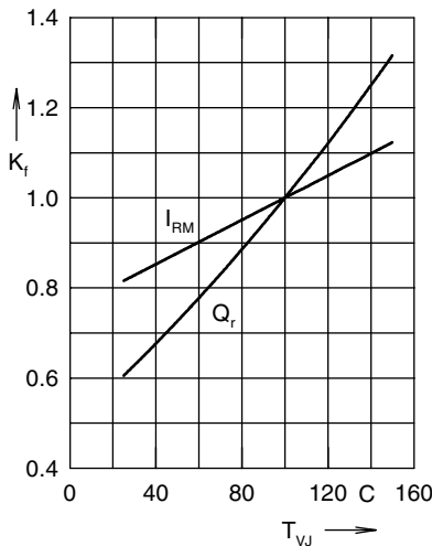
Fig. 4 Dynamic parameters K_f , I_{RM} , Q_r versus T_{VJ}
