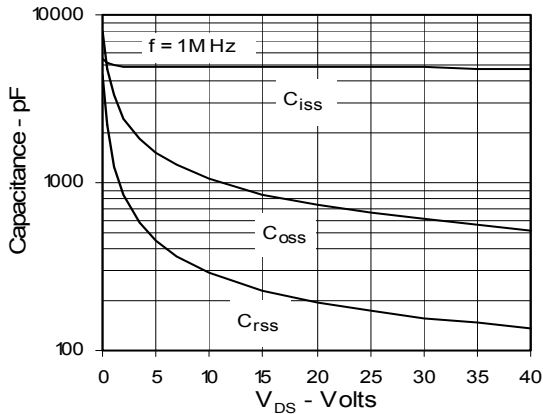
Fig. 11. Capacitance
