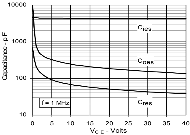
Fig. 9. Capacitance
