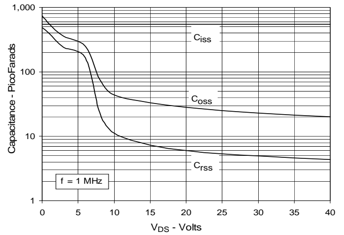
Fig. 10. Capacitance
