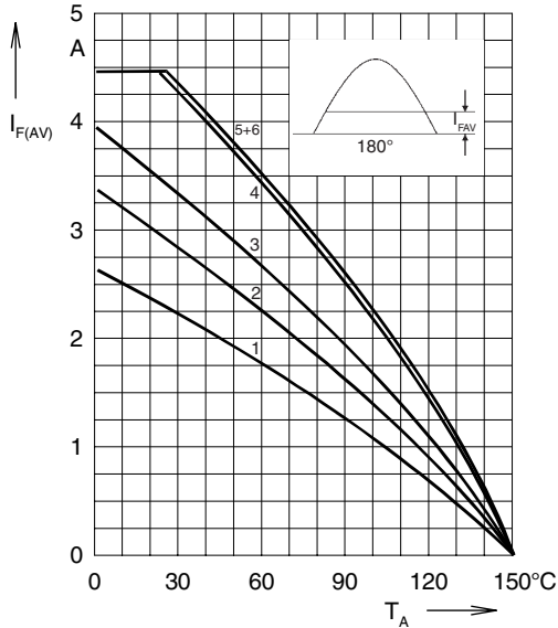
Fig. 4: Load diagramm
