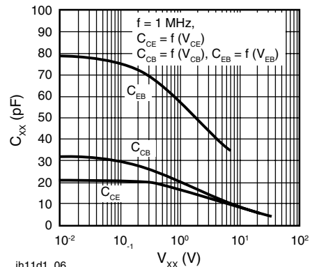
Fig. 5 - Transistor Capacitances (Typ.)
