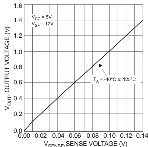
Fig. 5 Output Voltage
