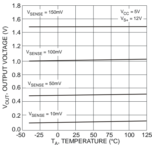
Fig. 6 Output Voltage
