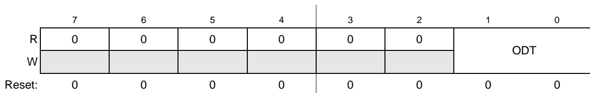
Figure 21. CPLD_SDODT Register
