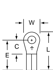
MU14-4R/S Stud Size: 4 Wire Range: 16-14
