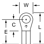
MU14-6R/S Stud Size: 6 Wire Range: 16-14
