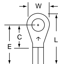
MU14-10R/L Stud Size: 10 Wire Range: 16-14
