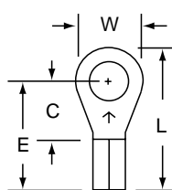
MU14-10R Stud Size: 10 Wire Range: 16-14
