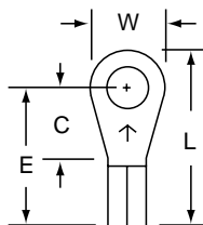
MU14-8R/L Stud Size: 8 Wire Range: 16-14
