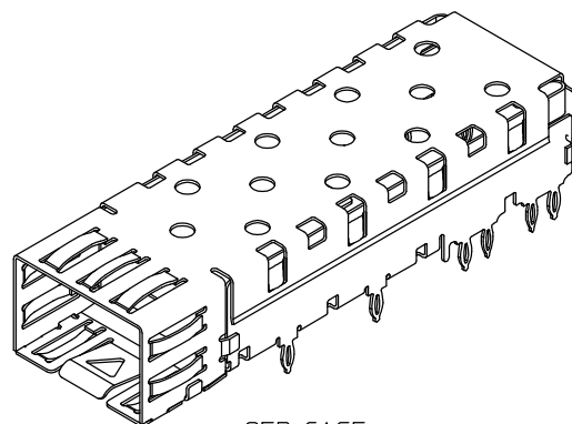
SFP CAGE SHOWN: 73927-0009
