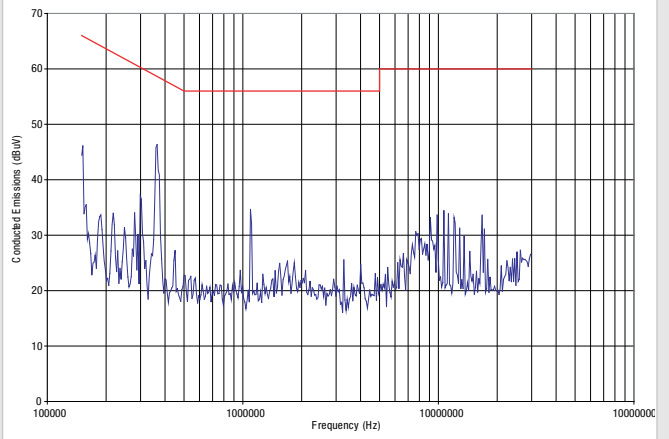
NPH25S2405
