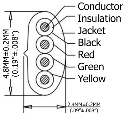
SEC:A-A
