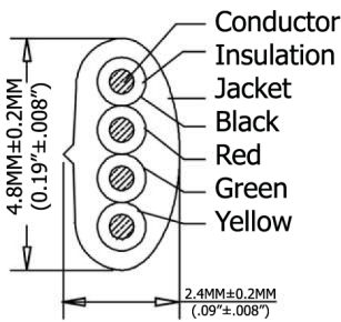
SEC:A-A
