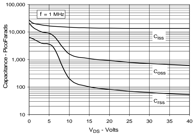
Fig. 11. Capacitance
