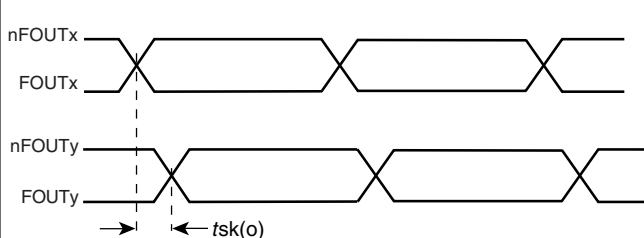
OUTPUT SKEW
