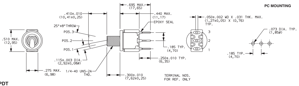
SPDT
