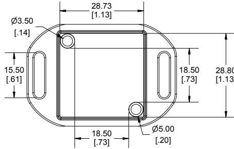
INSIDE LID
