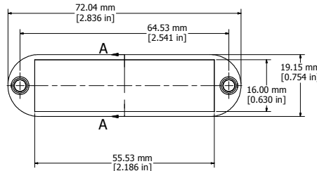
BEZEL
