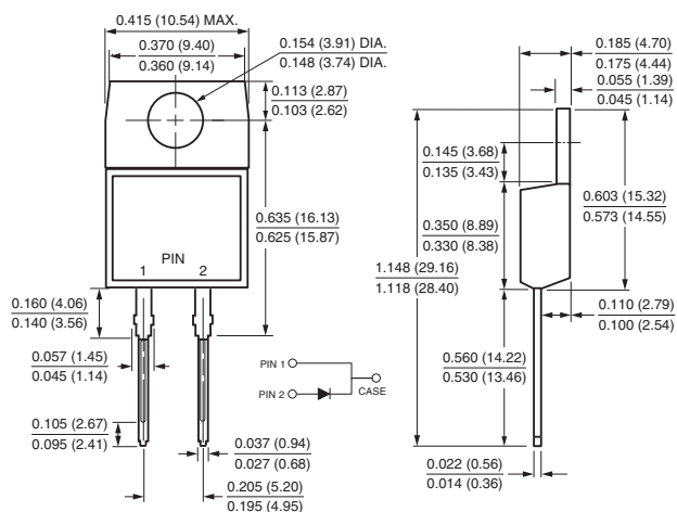
TO-220AC
