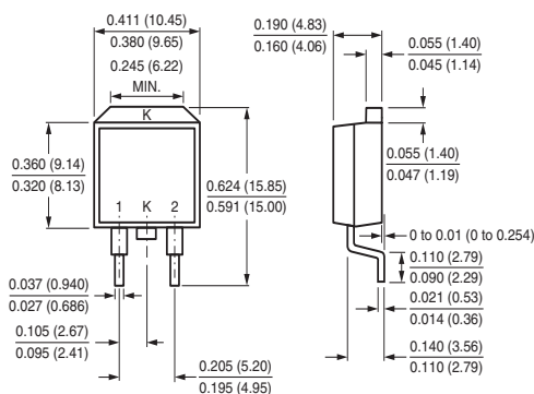
TO-263AB
