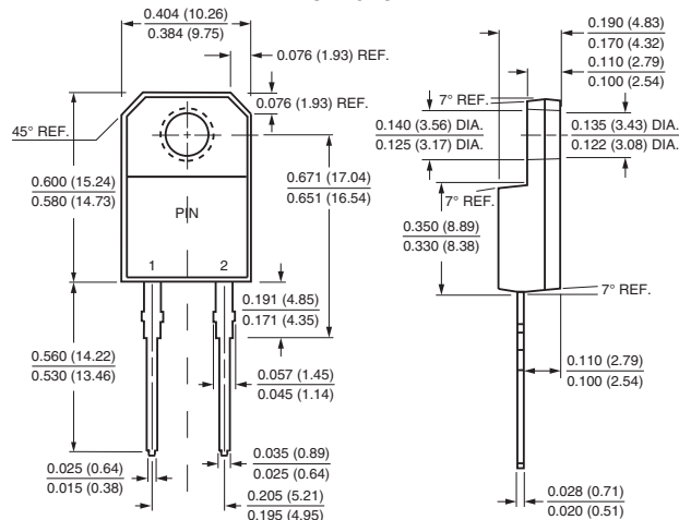
ITO-220AC
