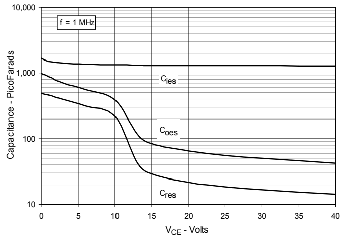
Fig. 10. Capacitance
