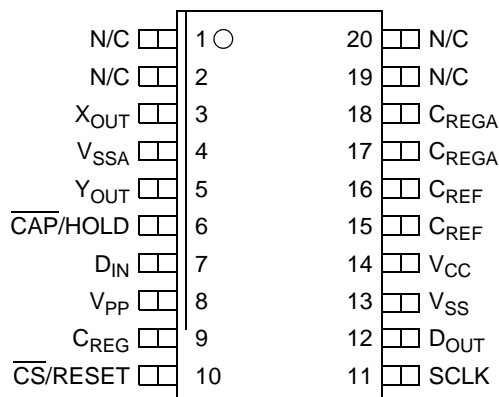
20-PIN SOIC PACKAGE
