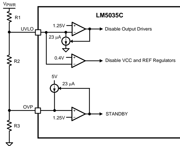
Figure 24. UVLO/OVP Divider
