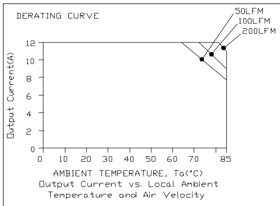
xRSB-40U02x, Vin=48V
