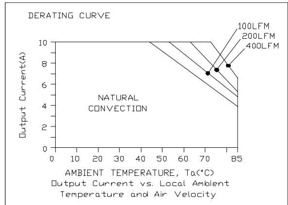
xRSB-40U03x, Vin=24V
