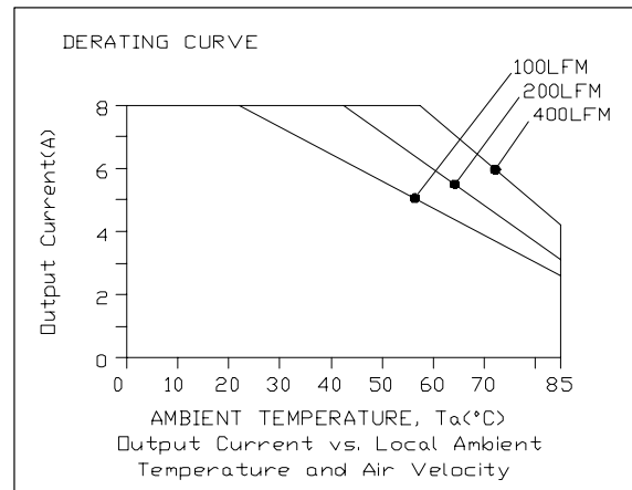
xRSB-40U05x, Vin=24V
