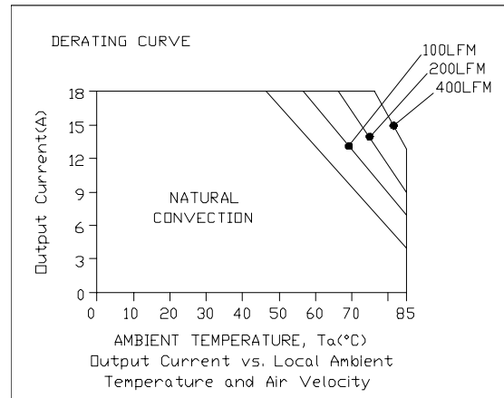
xRSB-40UV2x, Vin=24V
