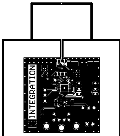
Top Layer
