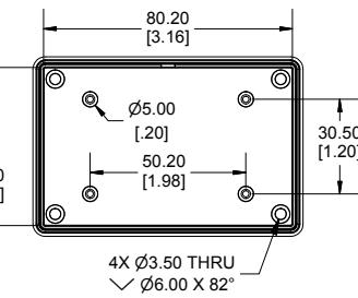
INSIDE LID
