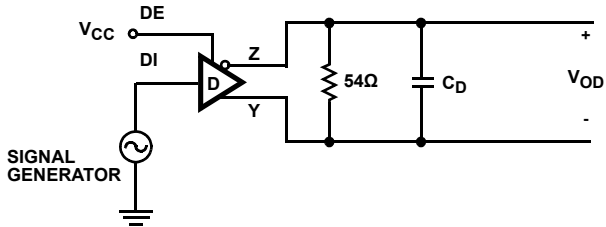
FIGURE 9A. TEST CIRCUIT
