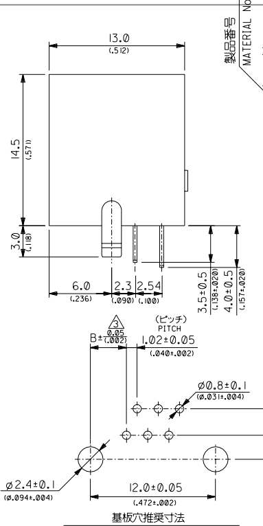
RECOMMENDED P.C.B. LAYOUT (ジャック取付け側) (JACK ASS'Y SIDE)
