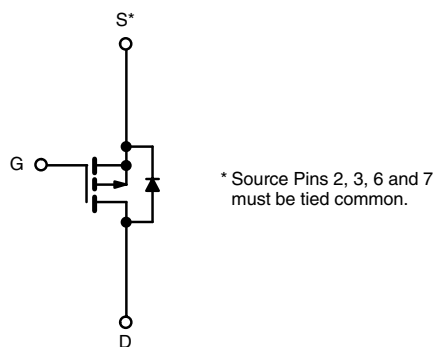
P-Channel MOSFET
