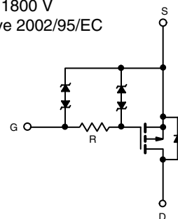
P-Channel MOSFET
