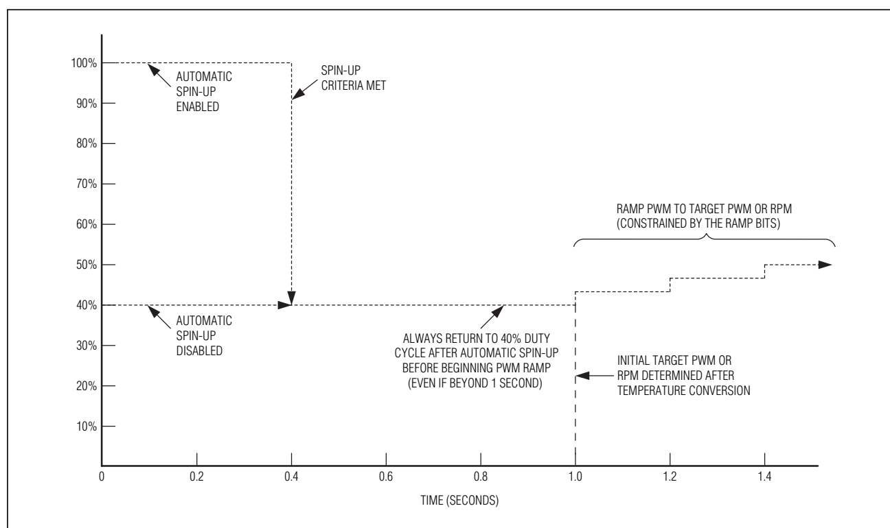
Figure 3. Fan Spin-Up
