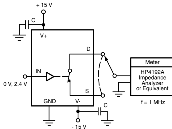
Fig. 6 - Capacitances
