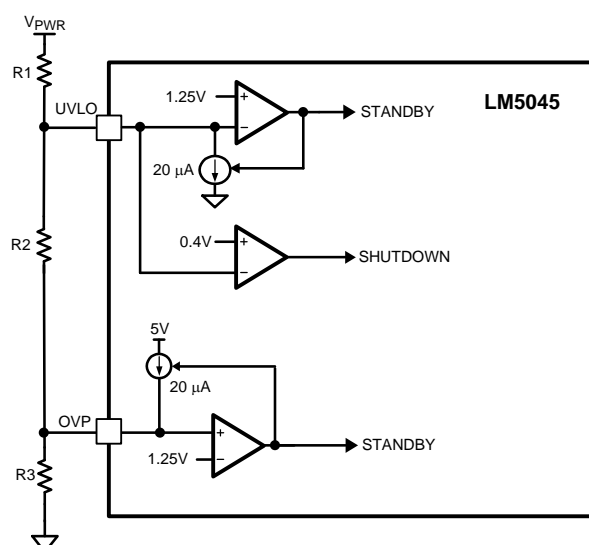
Figure 24. UVLO/OVP Divider
