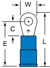
MNG14-4R/S Stud Size 4 Wire Range 16-14
