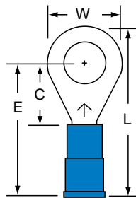
MNG14-14R/S Stud Size 1/4 Wire Range 16-14
