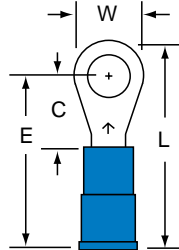
MNG14-10R/L Stud Size 10 Wire Range 16-14
