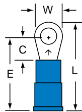
MNG14-6R/S Stud Size 6 Wire Range 16-14
