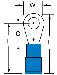
MNG14-8R/L Stud Size 8 Wire Range 16-14
