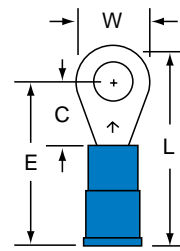
MNG14-8R Stud Size 8 Wire Range 16-14
