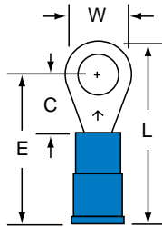
MNG14-10R Stud Size 10 Wire Range 16-14
