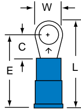
MNG14-8R/S Stud Size 8 Wire Range 16-14
