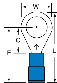
MNG14-516R/S Stud Size 5/16 Wire Range 16-14
