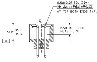
SECTION G-G SCALE - 4 : 1
