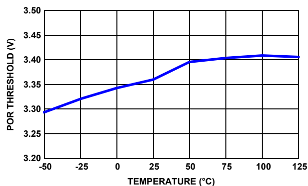
FIGURE 27. INPUT VOLTAGE POR THRESHOLD vs TEMPERATURE
