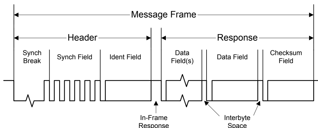
Figure 14-4. LIN Message
