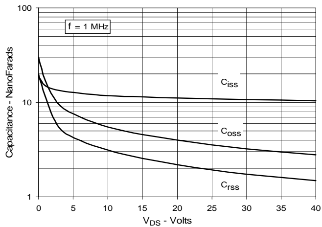
Fig. 11. Capacitance
