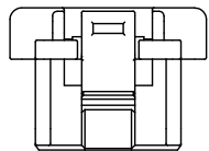
10CKTのロック形状 FIGURE OF 10 CIRCUIT
