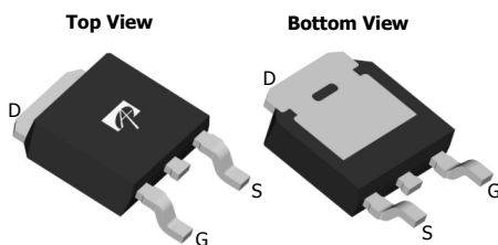
TO252 DPAK
