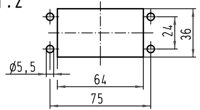
Montageausschnitt/ panel cut out 1:2
