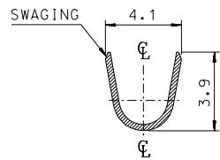
SEC' : C-C"
