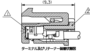
ターミナル及びリテーナー 接合状態概図 TERMINAL & RETAINER ASSEMBLY DRAWING
