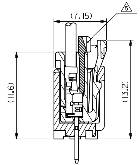
嵌合断面図
