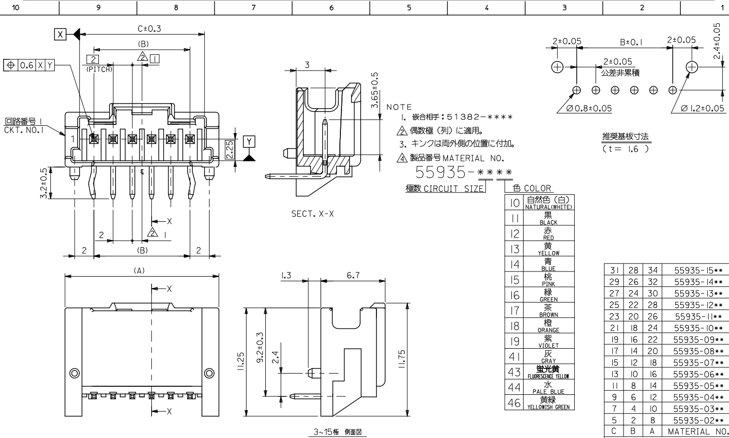
3~15極 側面図
