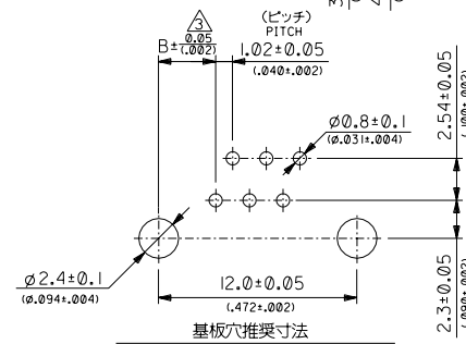
RECOMMENDED P.C.B. LAYOUT (ジャック取付け側) (JACK ASS'Y SIDE)
